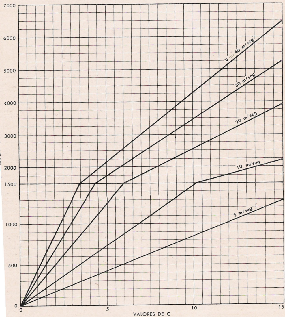
Gráfico 5: COEFICIENTE DE CONVECCION FORZADA DE VAPOR SOBREALENTADO CIRCULANDO DENTRO DE TUBOS
